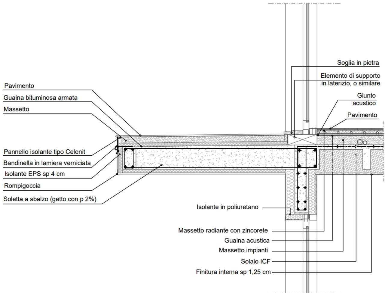
Figura 4.3 - Particolare del nodo balcone-solaio-parete-infisso. Notare la coibentazione che avvolge completamente la soletta del balcone e le modalità di aggancio dell'infisso, con completa eliminazione dei ponti termici.
